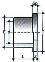
L Longitud campana E Diámetro externo Sp Espesor
