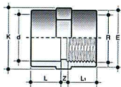
R Diámetro rosca L Longitud campana L1 Longitud rosca
