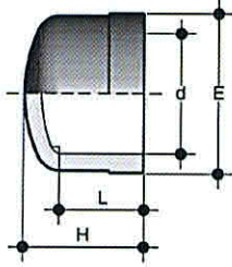
d Diámetro nominal L Longitud campana H Longitud total E Diámetro externo
