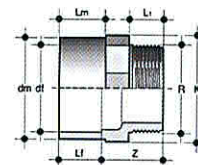
dm diámetro mayor R Diámetro rosca Lf Longitud campana L1 Longitud rosca dn Diámetro mayor dn Diámetro menor
